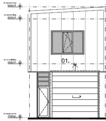
VORGEVEL 01. buitenverlichting
