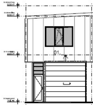
VORGEVEL 01. buitenverlichting
