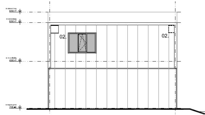
ZIJGEVEL 02. vloermuiskast
