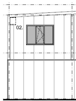
ACHTERGEVEL 02. vloermuiskast
