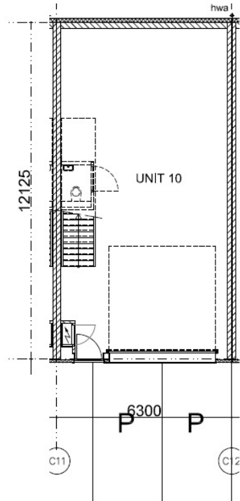
BEGANE GROND
