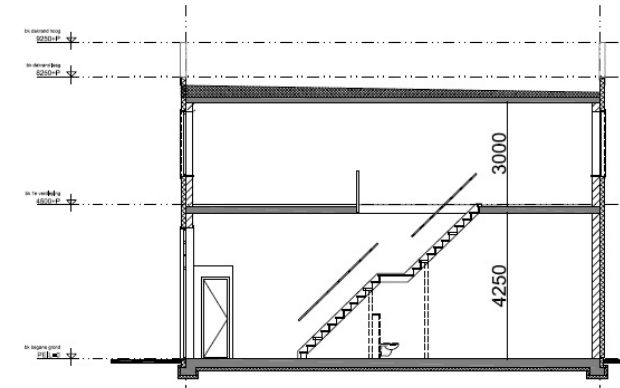
DOORSNEDE
