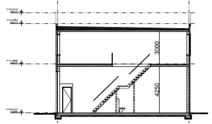
DOORSNEDE
