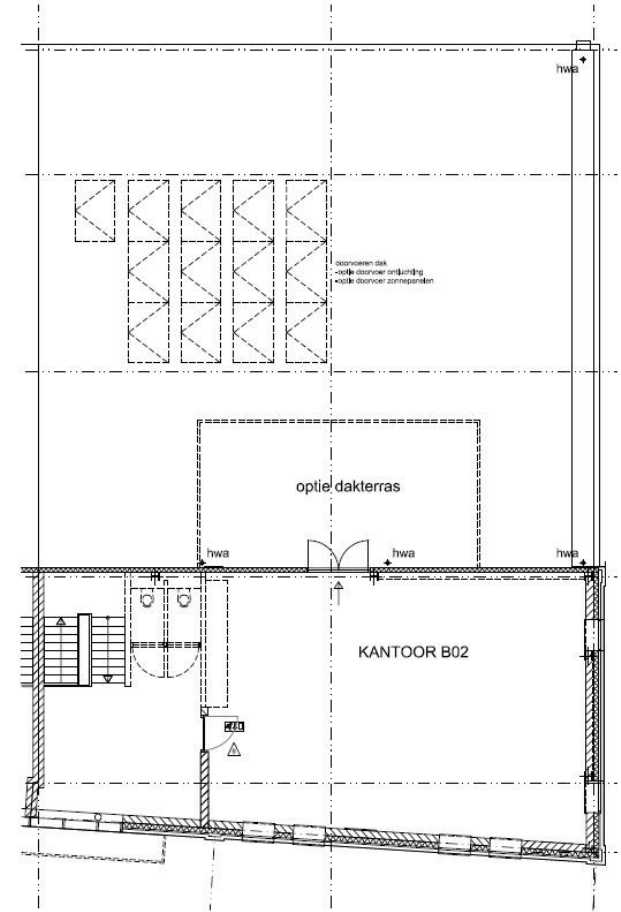
2e VERDIEPING
