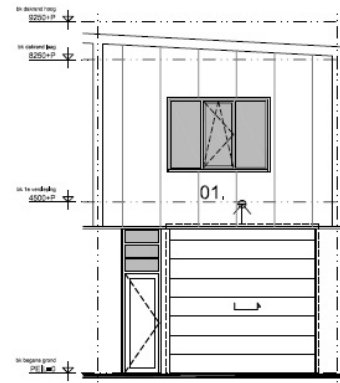
VOORGEVEL 01. buitenverlichting
