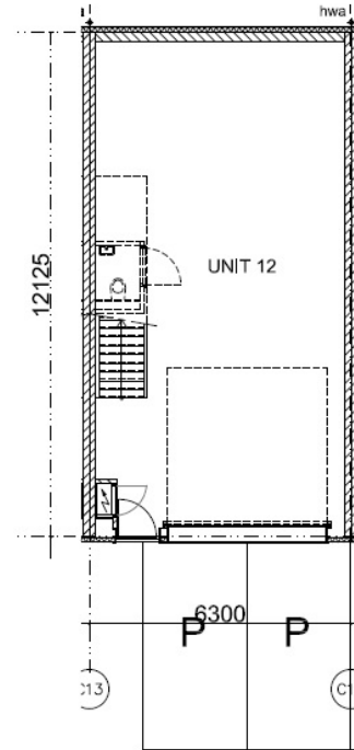
BEGANE GROND
