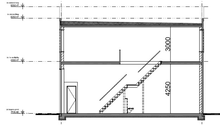
DOORSNEDE
