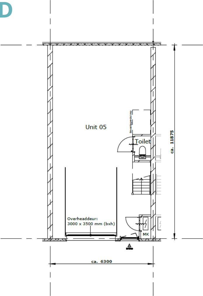
■ Begane Grond
