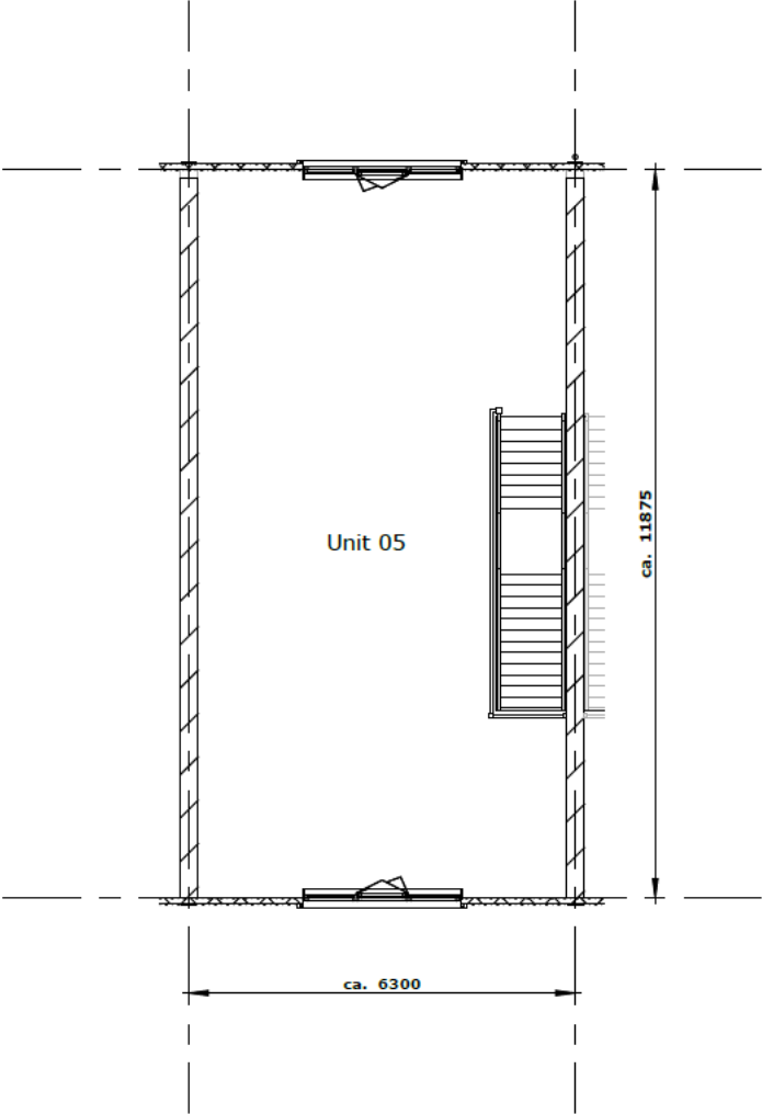
■ Eerste Verdieping
