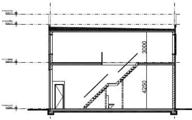
DOORSNEDE
