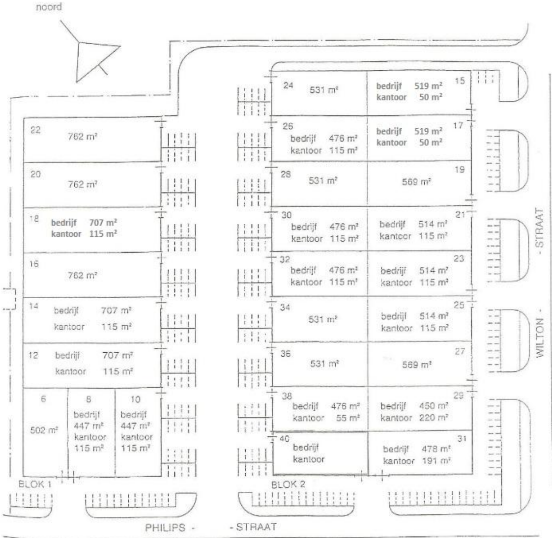
SITUATIE
